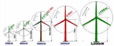
図 14 従来の風車と 3,000kW 風車の代表的寸法
