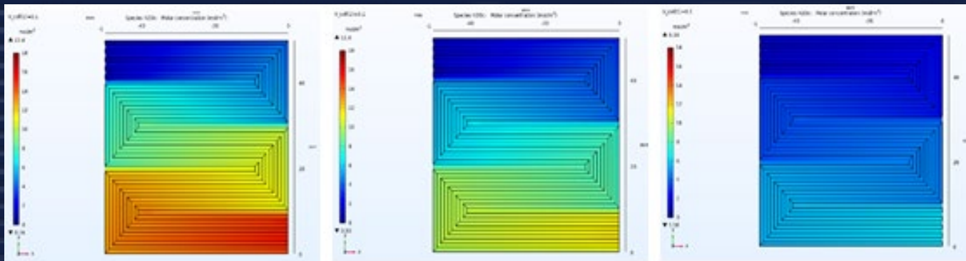
燃料電池内部の水蒸気濃度分布(数値解析結果)
