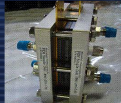
単セル内部温度分布 測定実験装置
